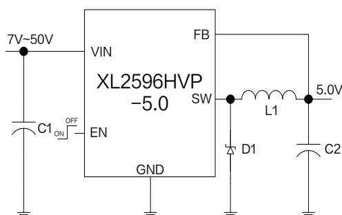
图1.XL2596HVP-5.0典型应用示意图和转换效率曲线
