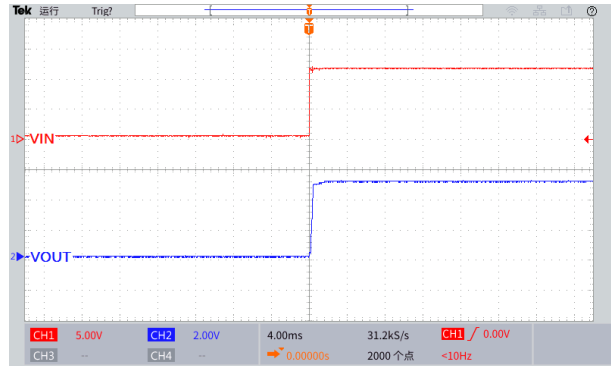
图 24.上电波形图
