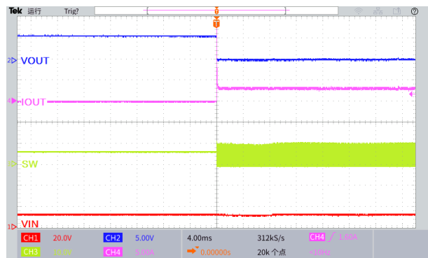
图 28.输出短路波形
