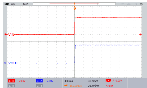
图 27.上电波形图
