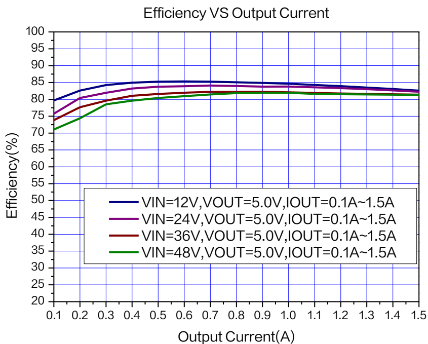
图 5. XL2596HVP -ADJ 系统效率曲线
