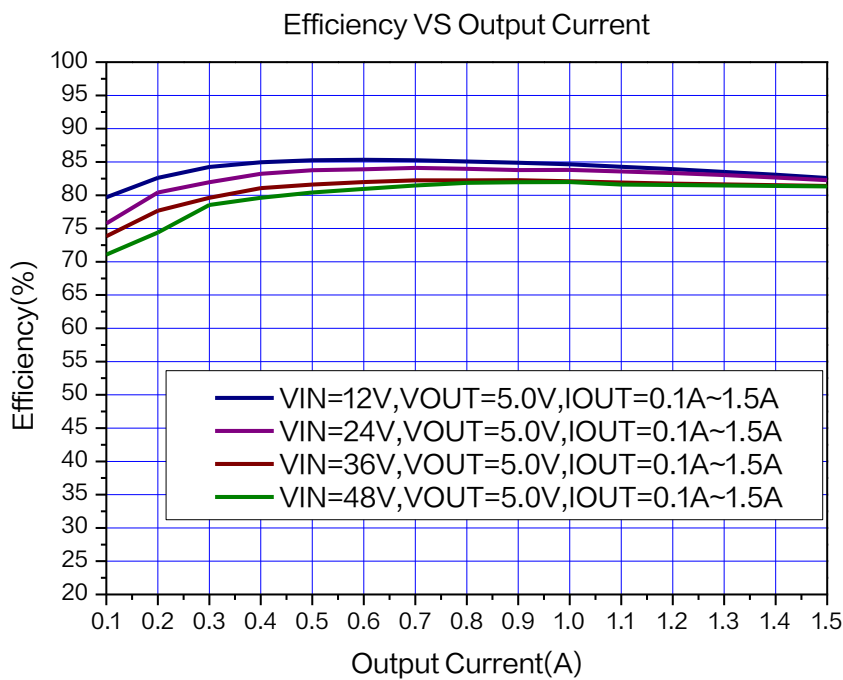
图 11. XL2596HVP-5.0 系统效率曲线
