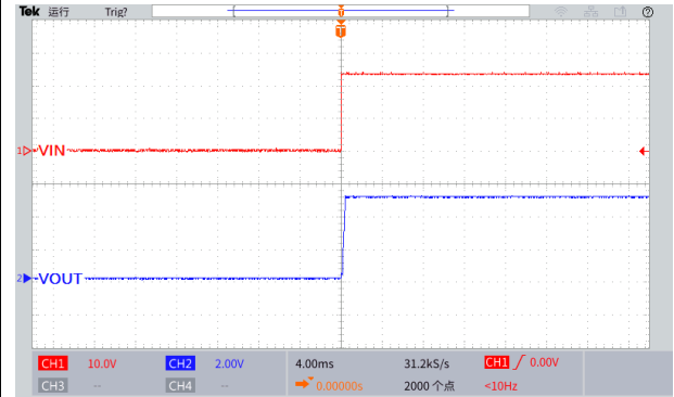
图 25.上电波形图
