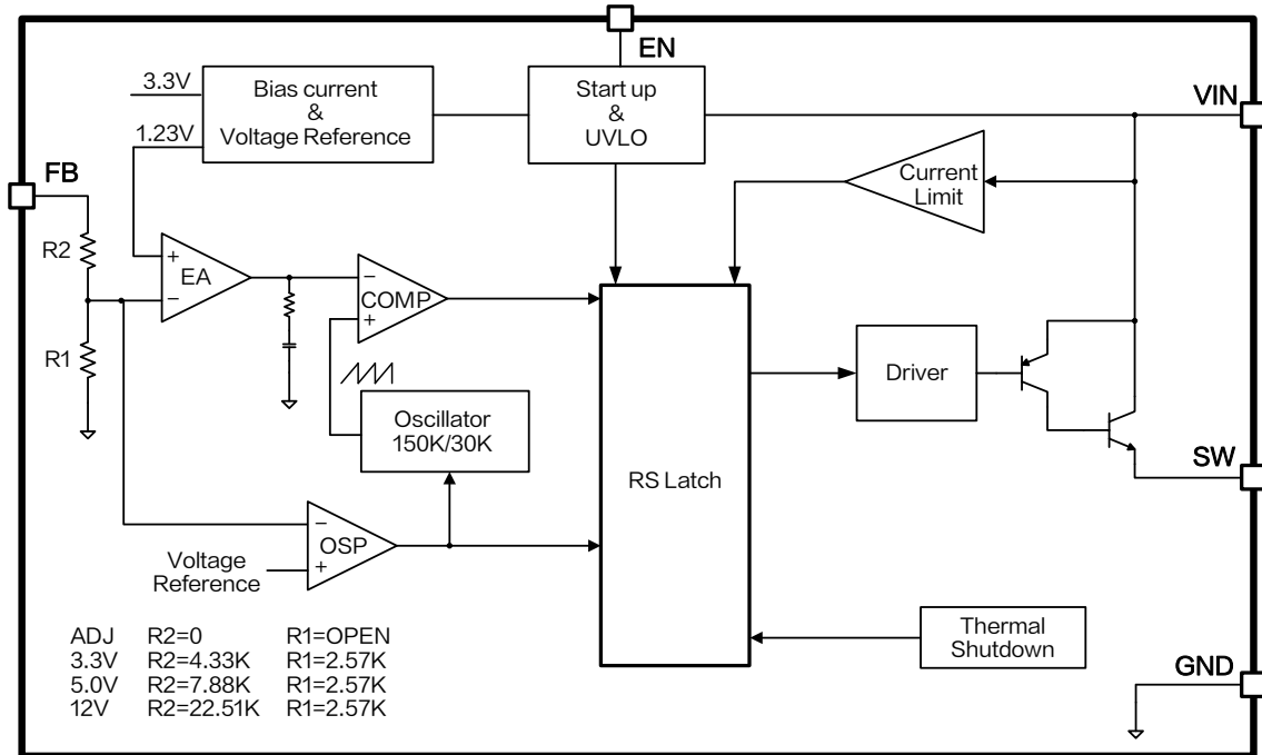
图 3. XL2596HVP 方框图
