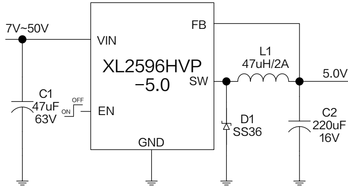
图 10.XL2596HVP-5.0 系统参数测量电路
