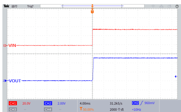
图 26.上电波形图
