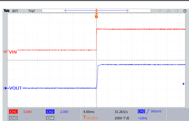
图 24.上电波形图
