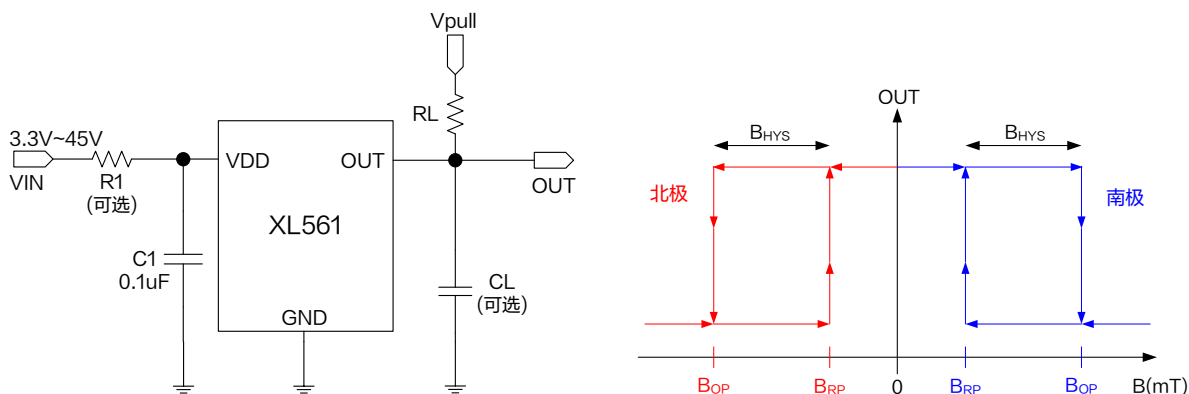
图 1. XL561 典型应用示意图和输出特性曲线
