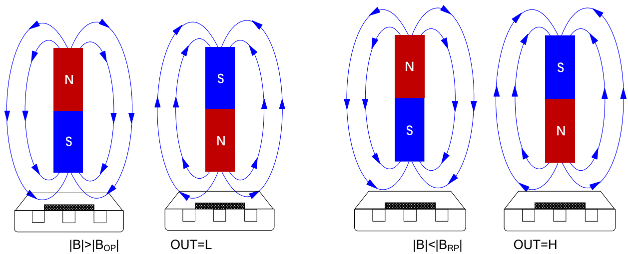
图 4. XL561 磁场方向定义图
