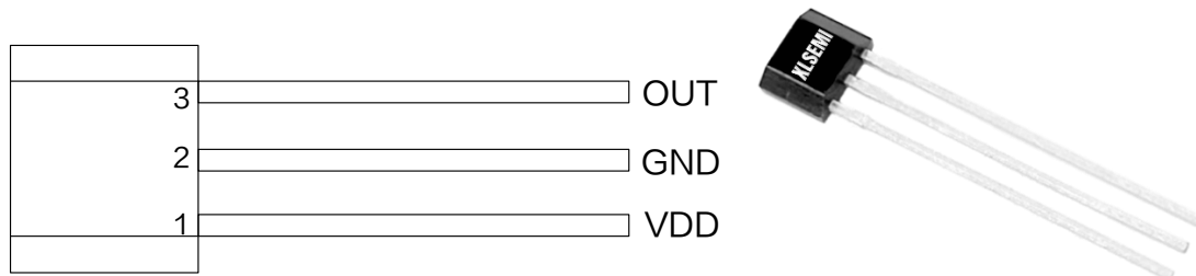
图 2. XL561 引脚配置
