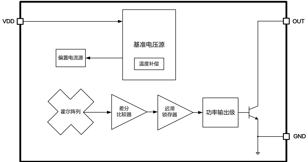
图 3. XL561 功能方框图
