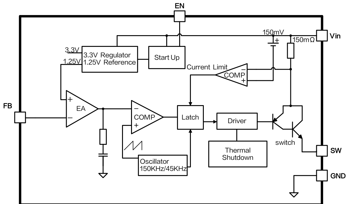
图 3. XL7005A 方框图
