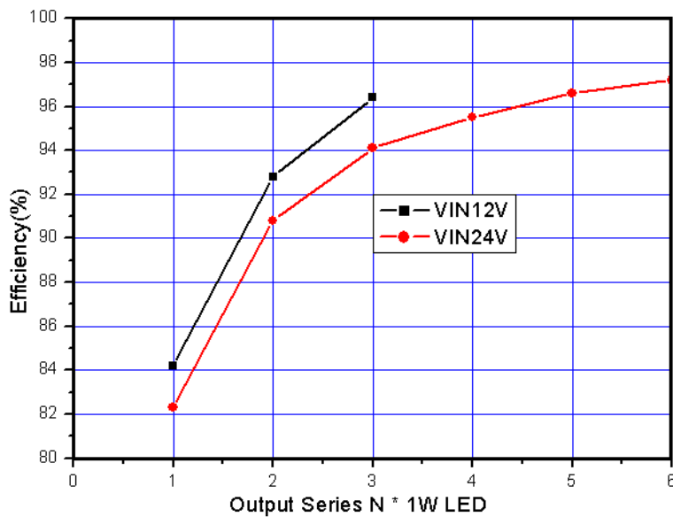
图12. XL8002系统效率曲线 (VIN=12V~36V)
