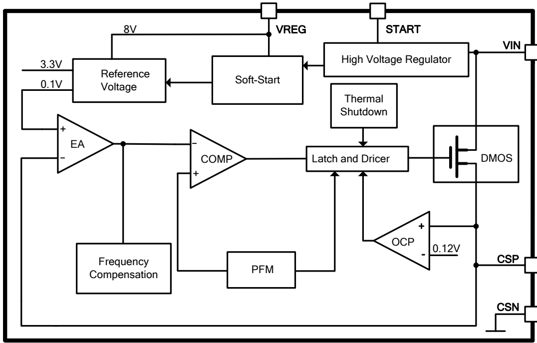
图 3. XL8002 方框图
