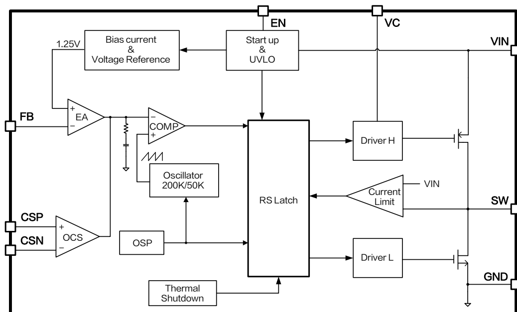
图 3. XL9009 方框图
