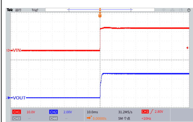
图 22.上电波形图
