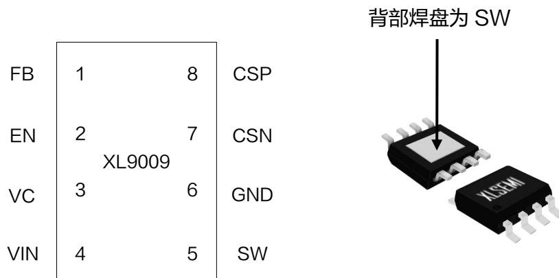
图 2. XL9009 引脚配置
