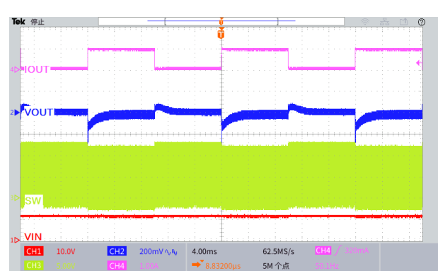
图 29.瞬态负载响应波形 ( V_{IN}=12V , V_{OUT}=5.0V , I_{OUT}=0.1 至 1A )
