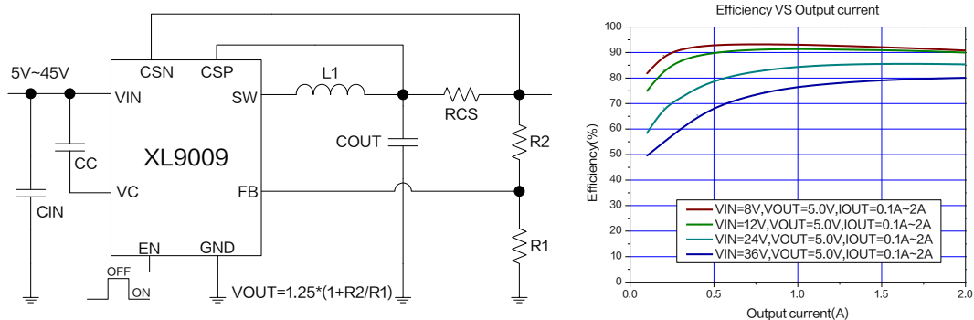
图1.XL9009典型应用示意图和转换效率曲线
