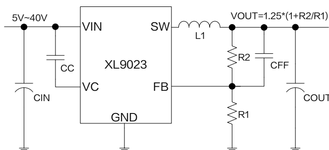
图1.XL9023典型应用示意图和转换效率曲线
