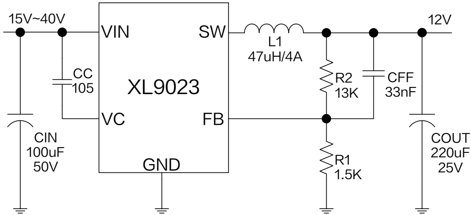
图 8. XL9023 系统参数测量电路 ( V_{IN}=15V\sim 40V, V_{OUT}=12V, I_{OUT}=0\sim 2.5A )
