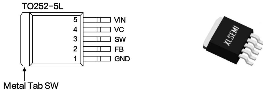
图 2. XL9023 引脚配置
