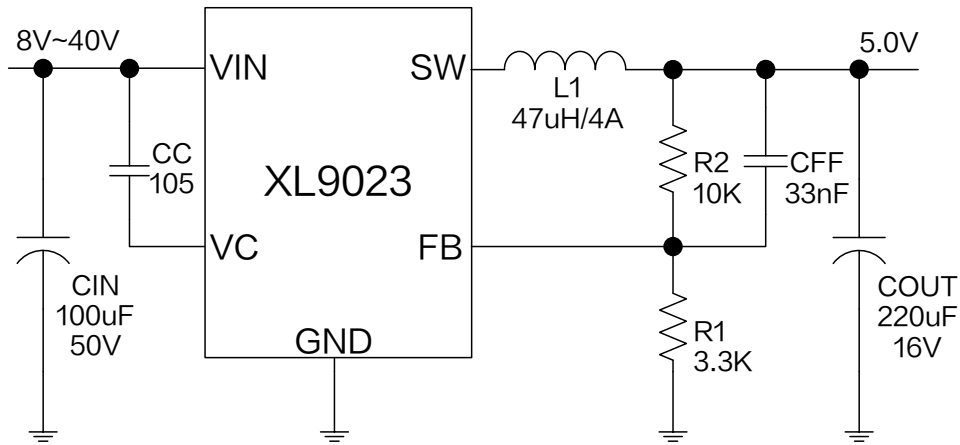
图 6. XL9023 系统参数测量电路 ( V_{IN}=8V\sim40V, V_{OUT}=5.0V, I_{OUT}=0\sim4A )
