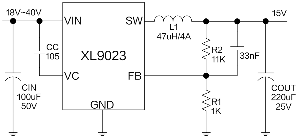
图 10. XL9023 系统参数测量电路 ( V_{IN}=18V\sim 40V, V_{OUT}=15V, I_{OUT}=0\sim 2A )
