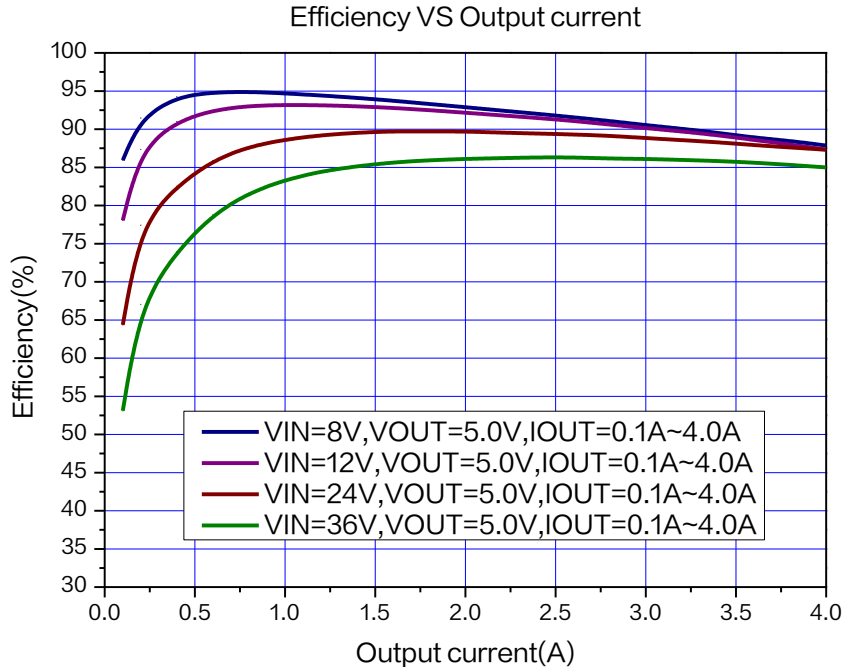
图 7. XL9023 系统效率曲线 ( V_{OUT}=5.0V )
