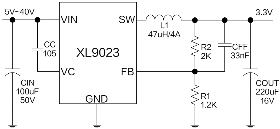
图 4. XL9023 系统参数测量电路 ( V_{IN}=5V\sim 40V, V_{OUT}=3.3V, I_{OUT}=0\sim 4A )
