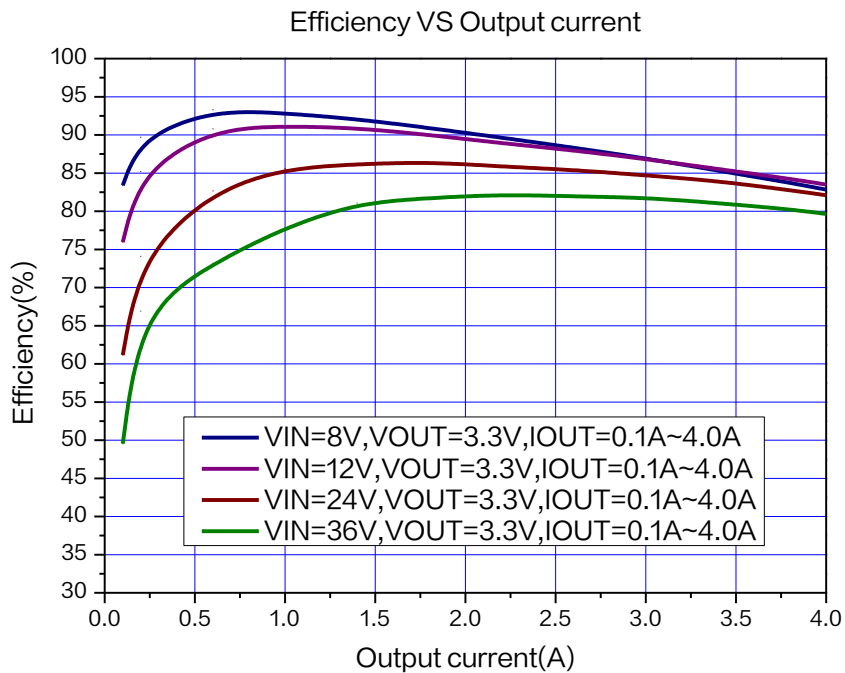
图 5. XL9023 系统效率曲线 ( V_{OUT}=3.3V )
