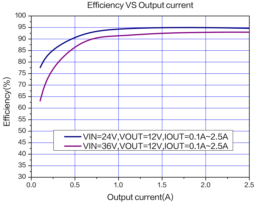
图 9. XL9023 系统效率曲线 ( V_{OUT}=12V )
