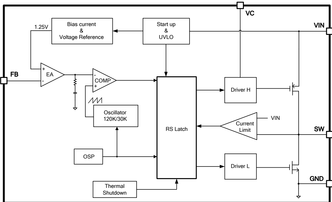
图 3. XL9023 方框图
