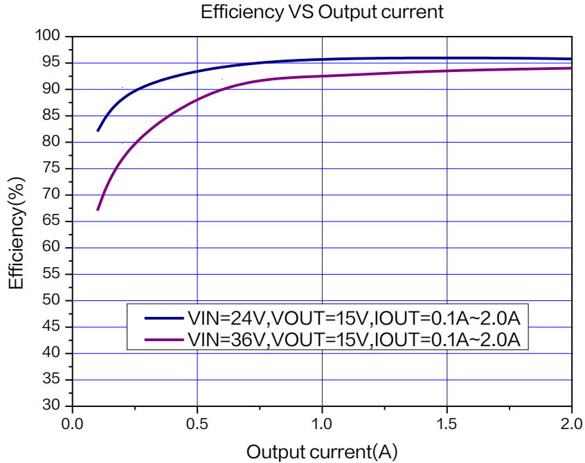
图 11. XL9023 系统效率曲线 ( V_{OUT}=15V )
