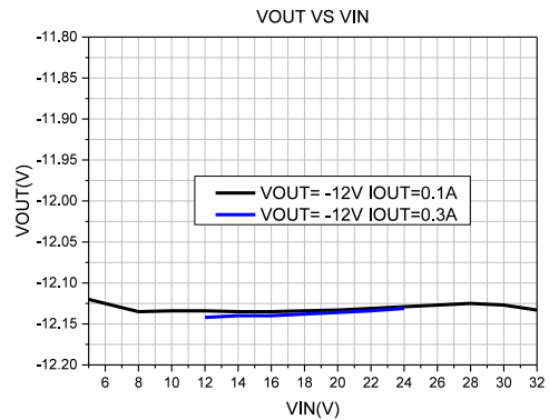
+12V 与 -12V 同时带载调整率
