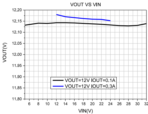
+12V 与 -12V 同时带载调整率
