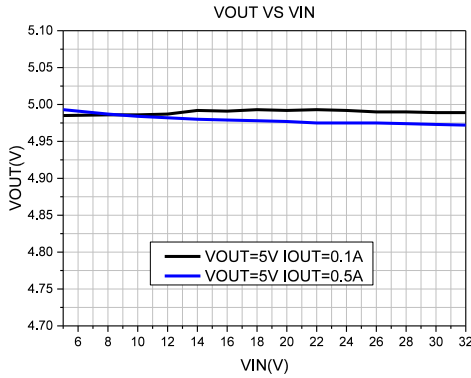
-5V 空载, +5V 带载调整率
