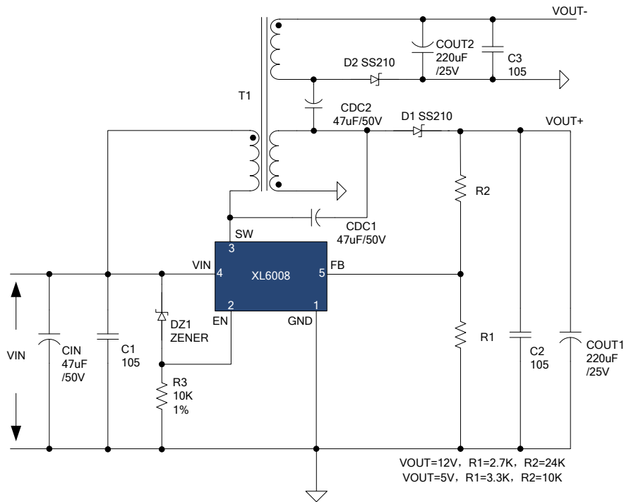
XL6008 正负压恒压方案原理图
