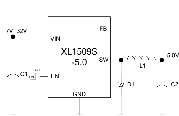
图1.XL1509S-5.0典型应用示意图和转换效率曲线
