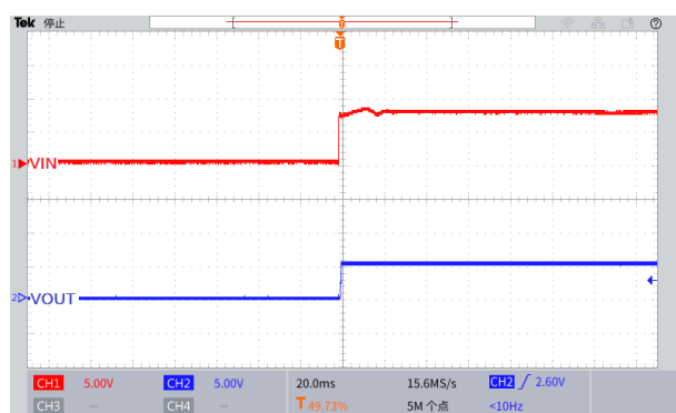
图 18.上电波形图 ( V_{IN}=8V , V_{OUT}=5.0V , I_{OUT}=0.1A )
