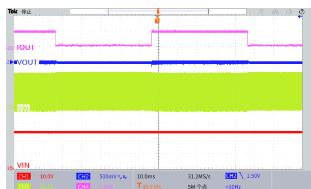
图 26.瞬态负载响应波形 ( V_{IN}=24V , V_{OUT}=5.0V , I_{OUT}=0.1 至 1A )
