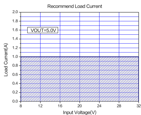
图 17.推荐输出电流 ( V_{OUT}=5.0V , T_A=25^{\circ}C )
