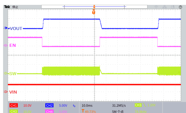
图 27. EN 引脚开关机波形 ( V_{IN}=8V , V_{OUT}=5.0V , I_{OUT}=0.5A )
