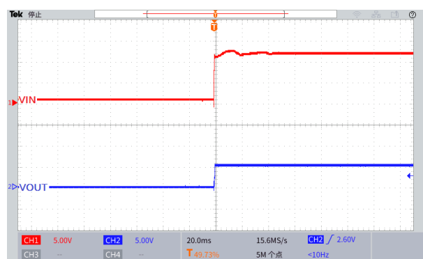
图 19.上电波形图 ( V_{IN}=12V , V_{OUT}=5.0V , I_{OUT}=0.1A )
