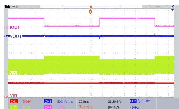
图 24.瞬态负载响应波形 ( V_{IN}=8V , V_{OUT}=5.0V , I_{OUT}=0.1 至 1A )
