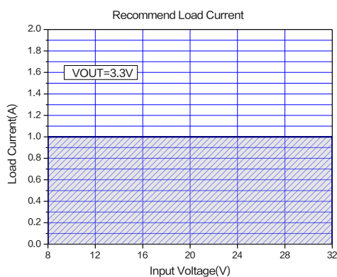
图 16.推荐输出电流 ( V_{OUT}=3.3V , T_A=25^{\circ}C )
