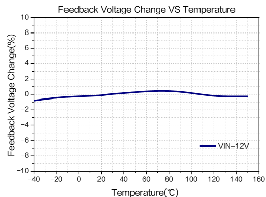
图 13.反馈电压温度系数曲线图
