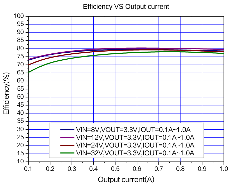
图 7. XL1509S-3.3 系统效率曲线
