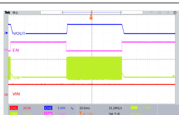
图 29.EN 引脚开关机波形 ( V_{IN}=24V , V_{OUT}=5.0V , I_{OUT}=0.5A )
