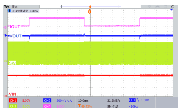
图 25.瞬态负载响应波形 ( V_{IN}=12V , V_{OUT}=5.0V , I_{OUT}=0.1 至 1A )
