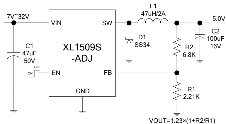
图 4. XL1509S-ADJ 系统参数测量电路 ( V_{OUT}=5.0V )
