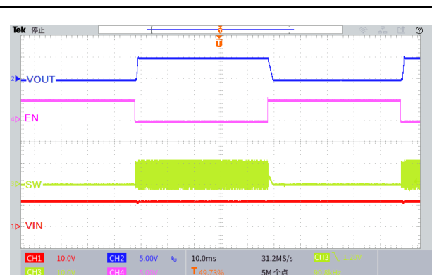
图 28.EN 引脚开关机波形 ( V_{IN}=12V , V_{OUT}=5.0V , I_{OUT}=0.5A )
