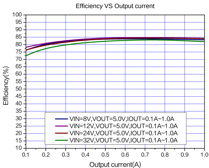
图 5. XL1509S-ADJ 系统效率曲线
