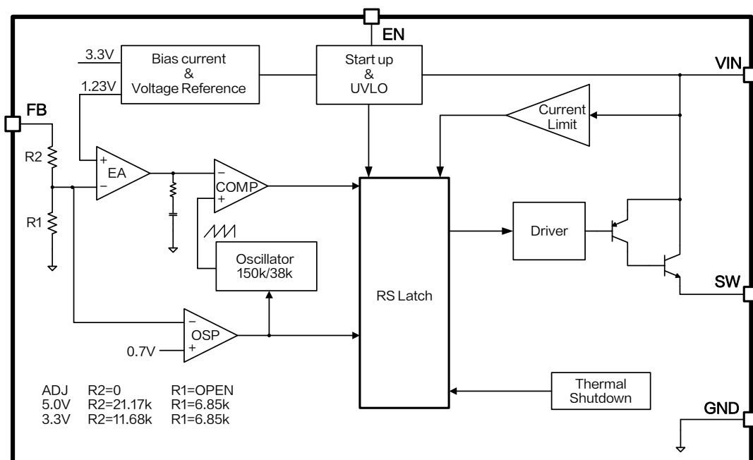
图 3. XL1509S 方框图
