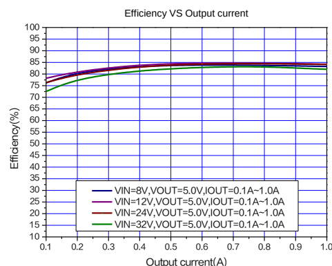
图1.XL1509S-5.0典型应用示意图和转换效率曲线
