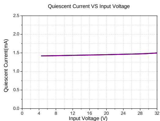
图 14. 静态电流曲线图
