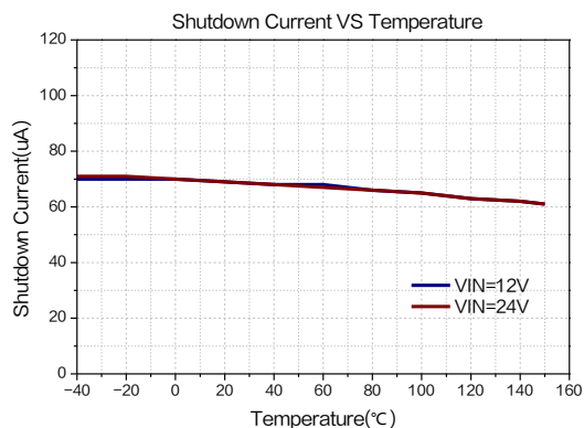
图 12. 关机电流温度系数曲线图
