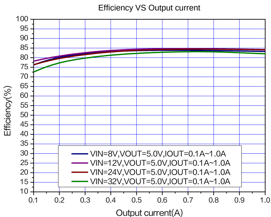
图 9. XL1509S-5.0 系统效率曲线
