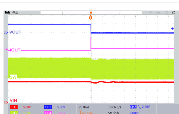
图 22.输出短路波形 ( V_{IN}=12V , V_{OUT}=5.0V )
