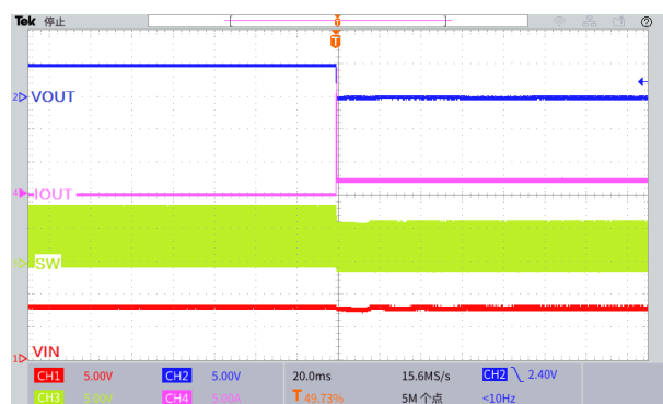
图 21. 输出短路波形 ( V_{IN}=8V , V_{OUT}=5.0V )
