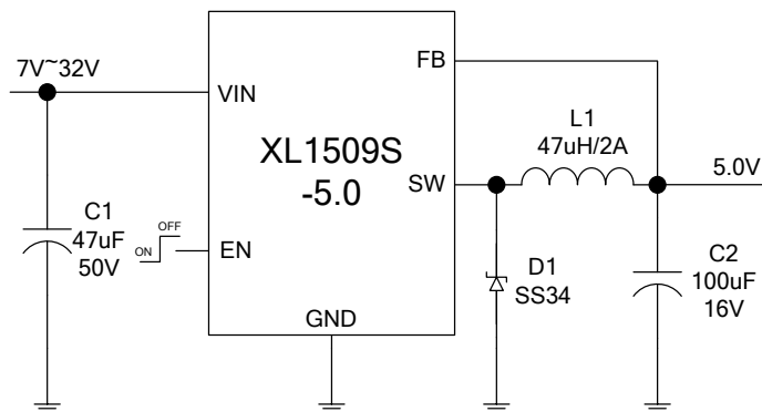
图 8.XL1509S-5.0 系统参数测量电路
