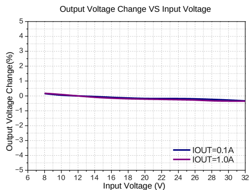
图 10.线性调整率曲线图
