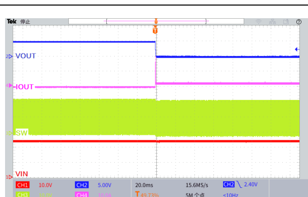
图 23.输出短路波形 ( V_{IN}=24V , V_{OUT}=5.0V )
