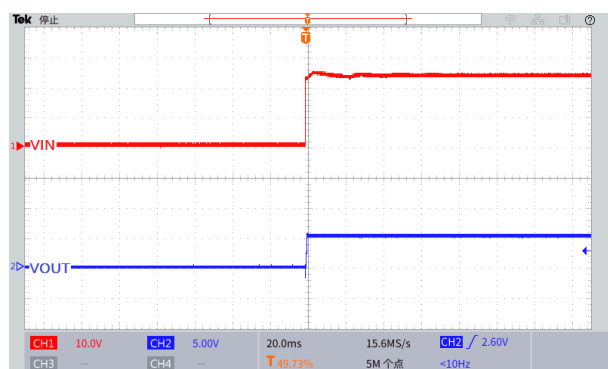
图 20.上电波形图 ( V_{IN}=24V , V_{OUT}=5.0V , I_{OUT}=0.1A )
