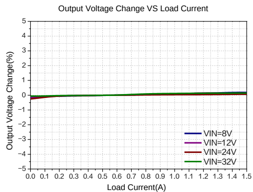
图 11.负载调整率曲线图
