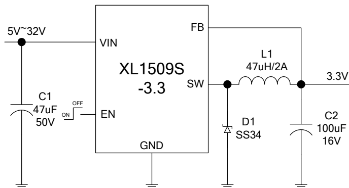
图 6.XL1509S-3.3 系统参数测量电路
