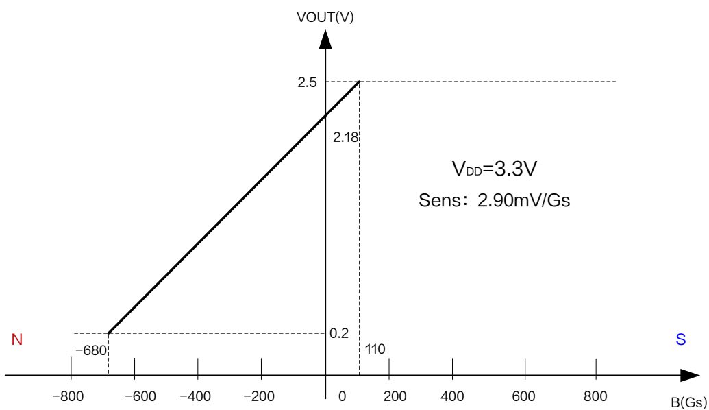
图 5.XL42N 输出特性曲线 ( V_{DD}=3.3V )
